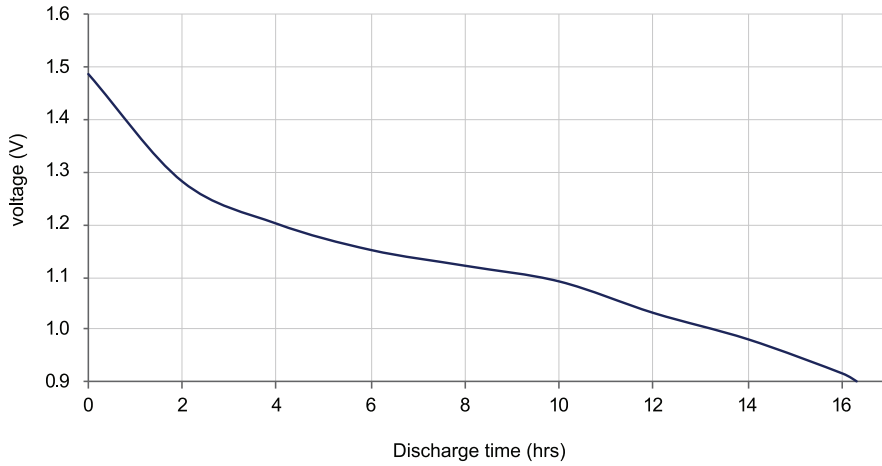
Portable Lighting 4m/15m 8h/d 2,2 ohm cutoff 0,9 V
