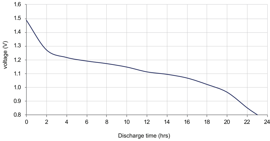
Portable stereo 2h/d 600 mA cutoff 0,9 V
